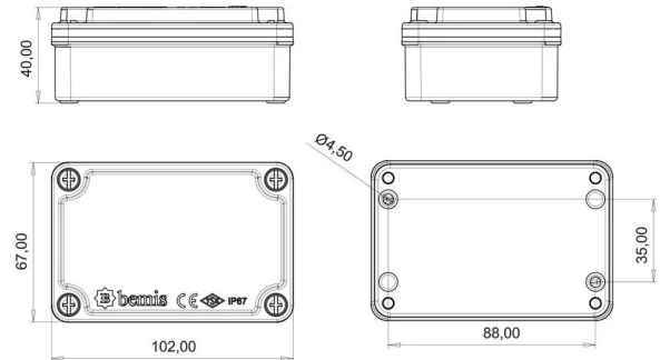
MASSZEICHNUNG
