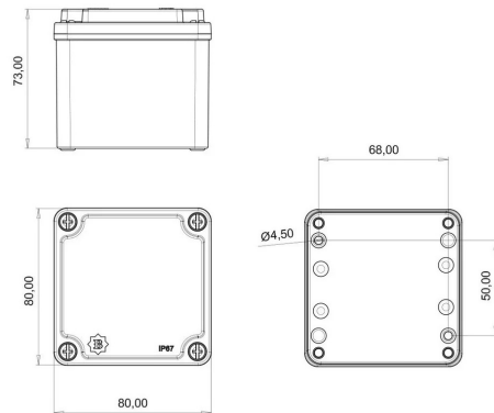
MASSZEICHNUNG
