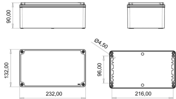
MASSZEICHNUNG
