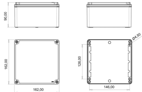
MASSZEICHNUNG
