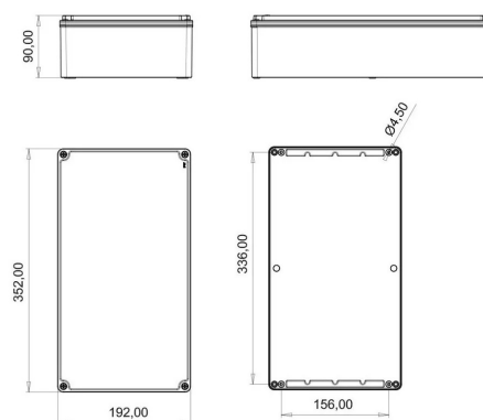
MASSZEICHNUNG
