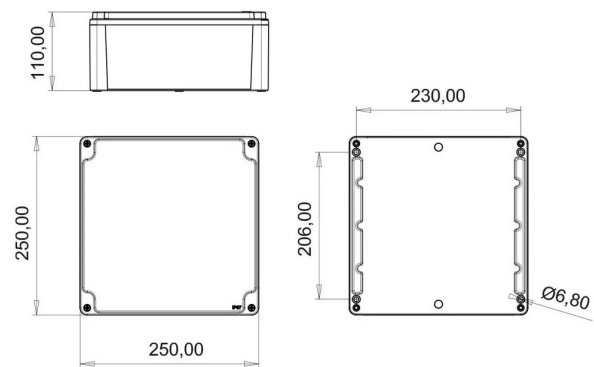
MASSZEICHNUNG
