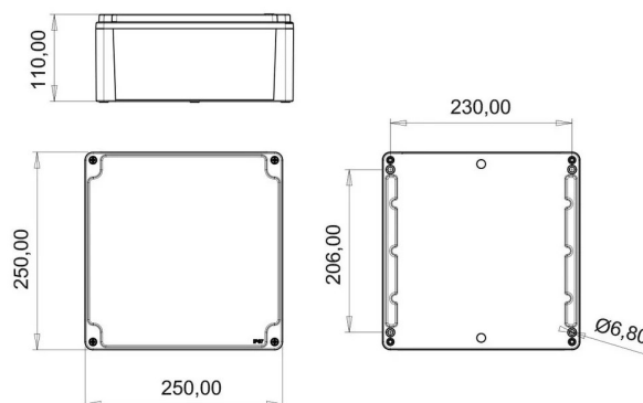
MASSZEICHNUNG
