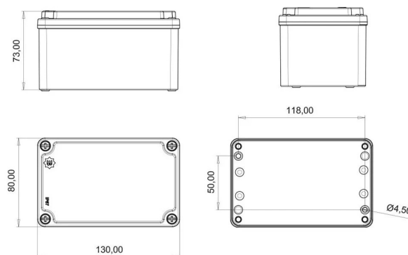
MASSZEICHNUNG
