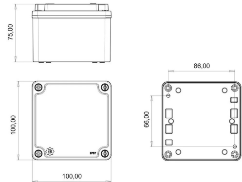
MASSZEICHNUNG
