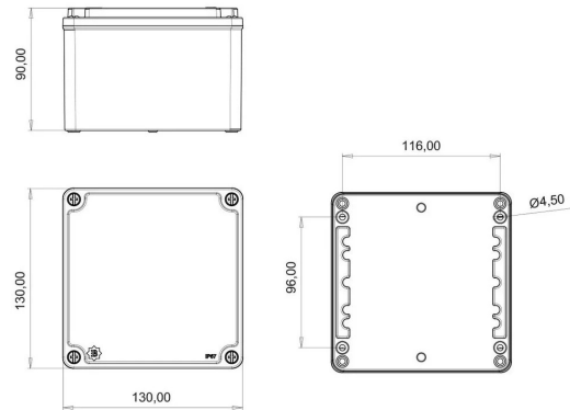
MASSZEICHNUNG
