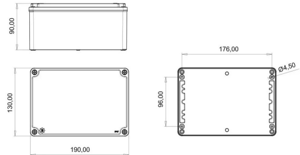
MASSZEICHNUNG
