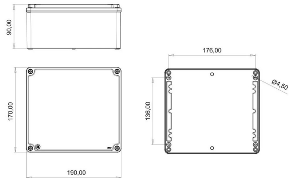
MASSZEICHNUNG
