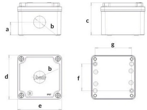
Ölçüler / Dimensions (mm)
