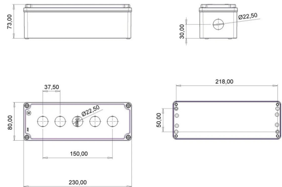
MASSZEICHNUNG
