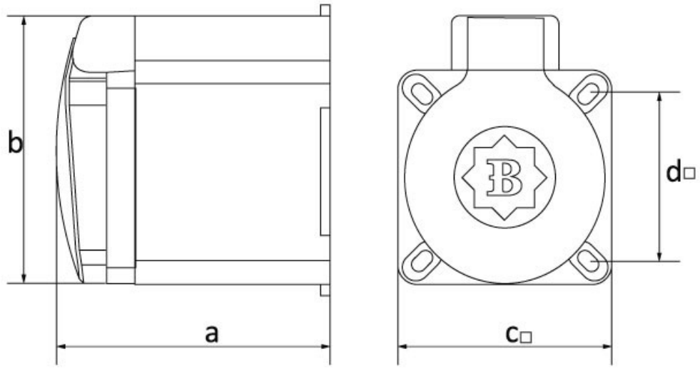
Ölçüler / Dimensions (mm)
