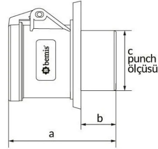
Ölçüler / Dimensions (mm)
