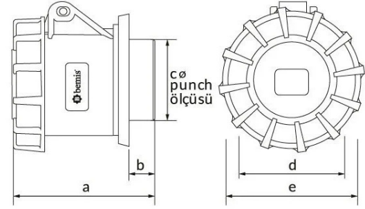
Ölçüler / Dimensions (mm)
