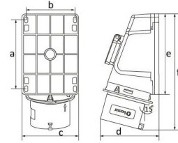
Ölçüler / Dimensions (mm)
