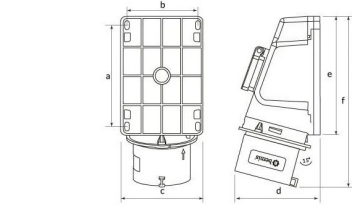
Ölçüler / Dimensions (mm)
