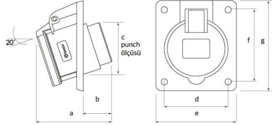
Ölçüler / Dimensions (mm)
