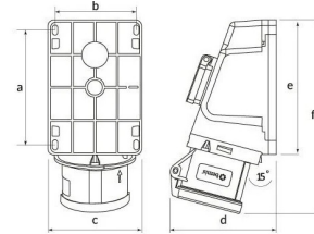
Ölçüler / Dimensions (mm)
