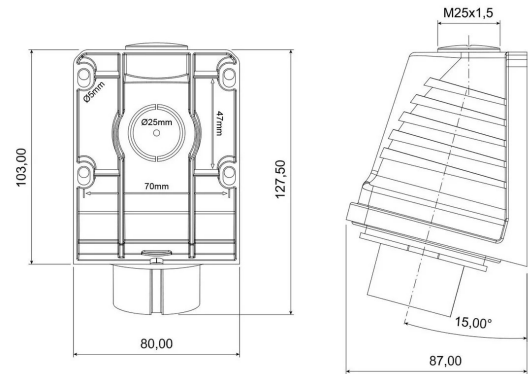
PLANO TÉCNICO
