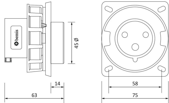
PLANO TÉCNICO
