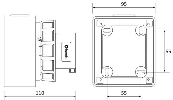
PLANO TÉCNICO
