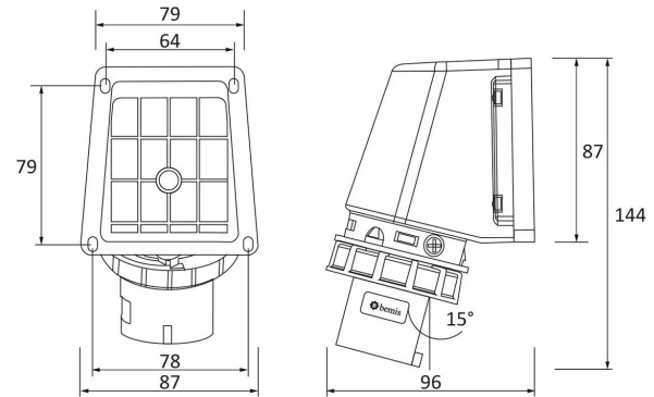
PLANO TÉCNICO
