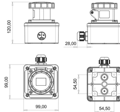
PLANO TÉCNICO
