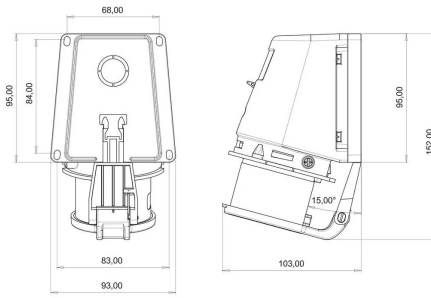
PLANO TÉCNICO
