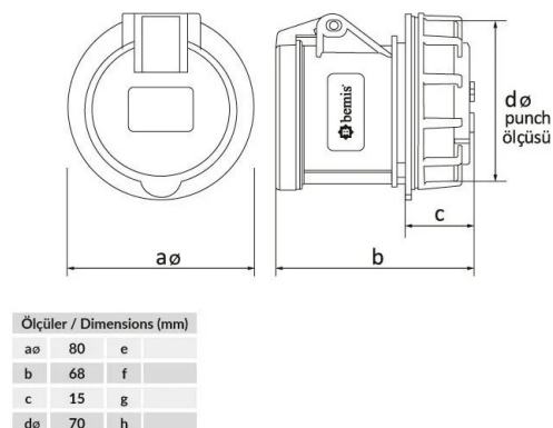
PLANO TÉCNICO
