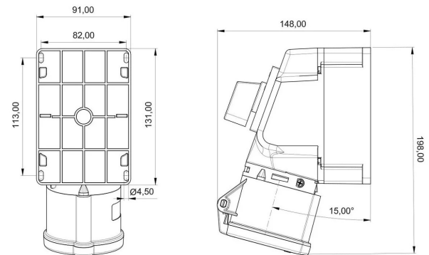
PLANO TÉCNICO
