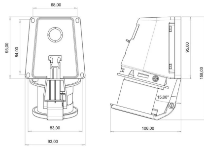
PLANO TÉCNICO
