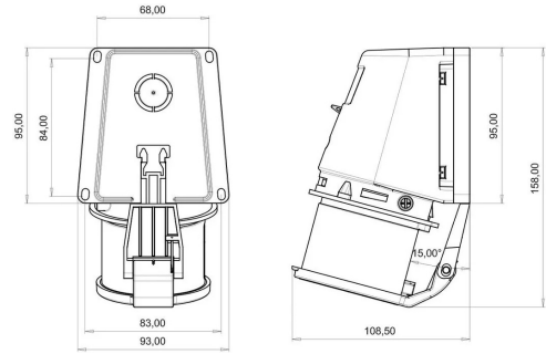
PLANO TÉCNICO
