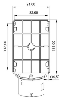
PLANO TÉCNICO
