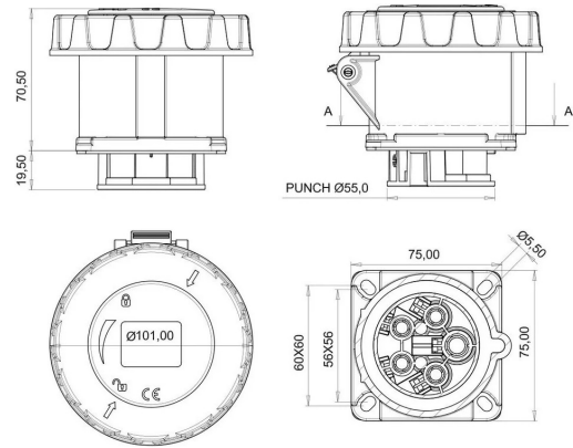
PLANO TÉCNICO
