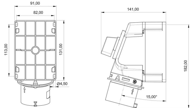
PLANO TÉCNICO
