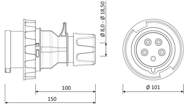
PLANO TÉCNICO
