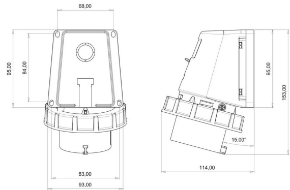
PLANO TÉCNICO
