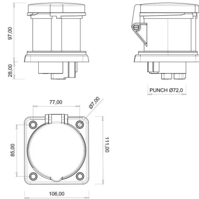
PLANO TÉCNICO
