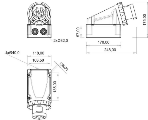
PLANO TÉCNICO
