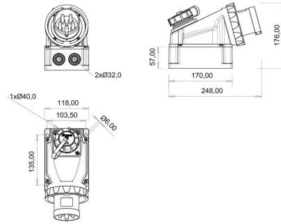
PLANO TÉCNICO
