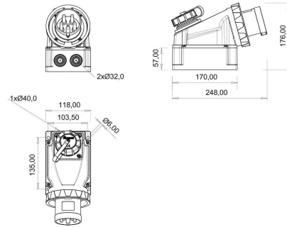
PLANO TÉCNICO
