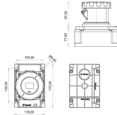
PLANO TÉCNICO
