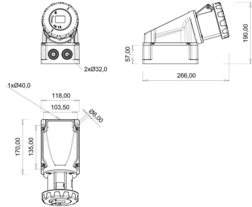
PLANO TÉCNICO
