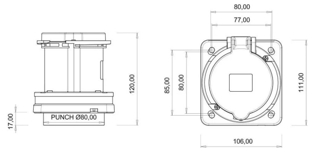
PLANO TÉCNICO
