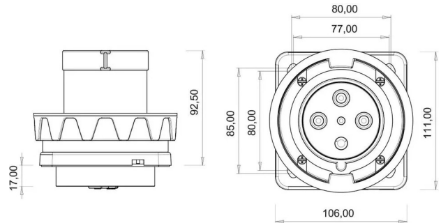
PLANO TÉCNICO
