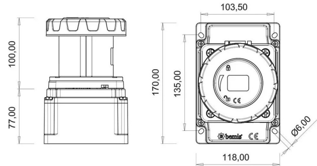
PLANO TÉCNICO
