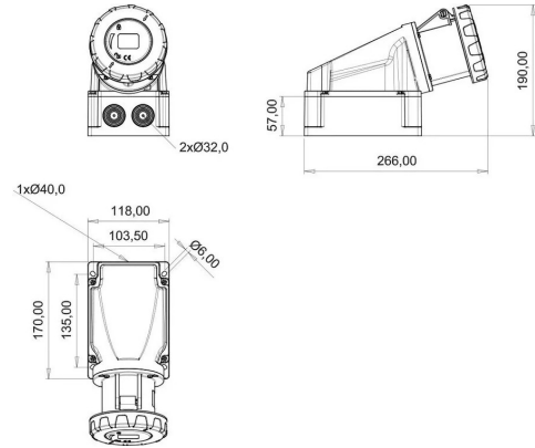
PLANO TÉCNICO
