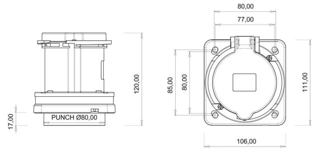
PLANO TÉCNICO
