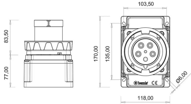
PLANO TÉCNICO
