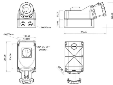
PLANO TÉCNICO
