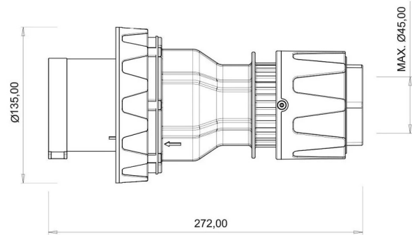
PLANO TÉCNICO
